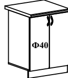
ШН 600 600x840x474
