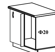
ШНУ 1000 1000x840x474
