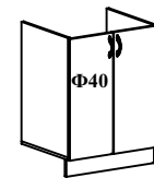
ШНМ 600 600x816x474
