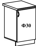
ШН 500 500x840x474
