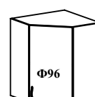
ШВУ 600 600x716x600
